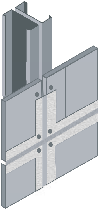
Juntas de control en muros.
