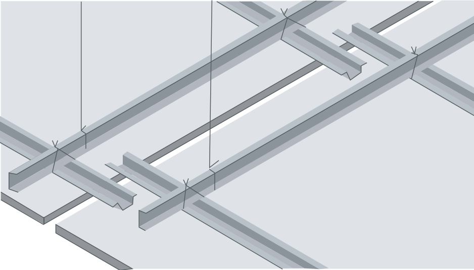
Juntas de control en plafón.
