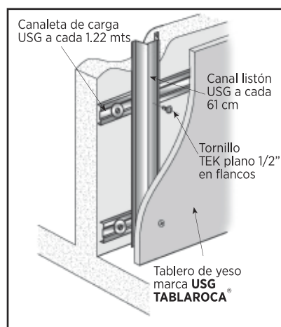
Lambrín a base de poste y canal
